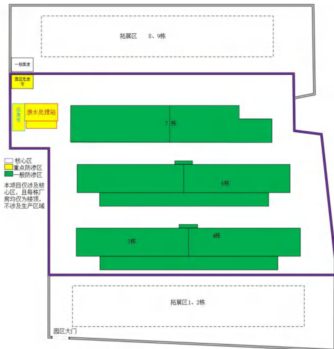
图 8.2-9 项目防渗分区图
