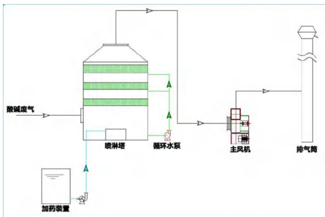
图 3.1-14 酸雾废气治理工艺流程图
