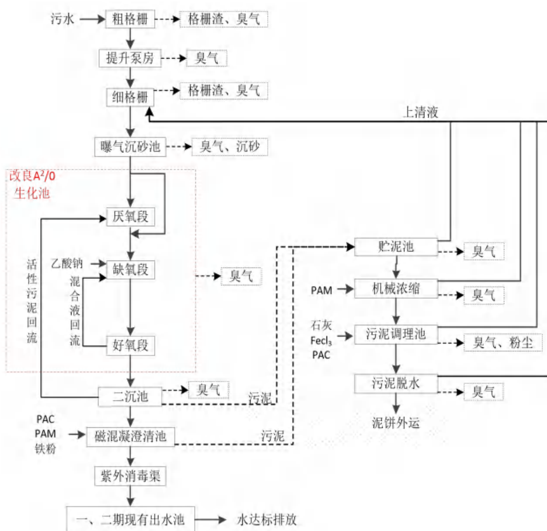
图 8.2-3 中山市阜沙镇污水处理有限公司三期污水处理工艺
