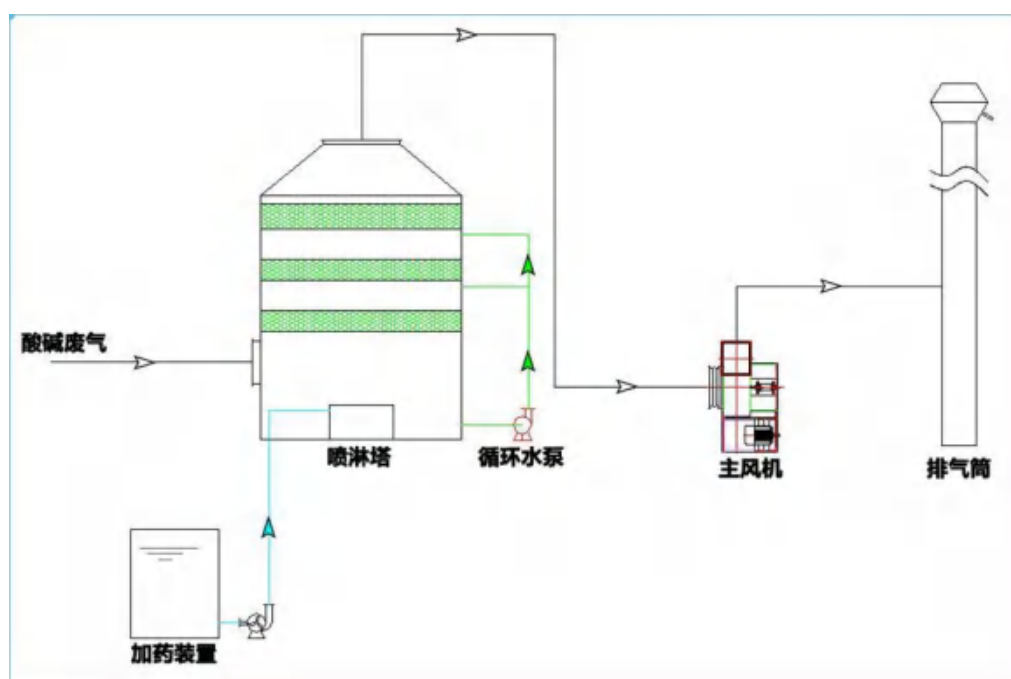
图 8.2-6 酸雾废气治理工艺流程图
