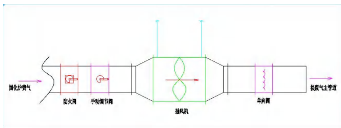
图 3.1-3 防倒灌措施示意图
