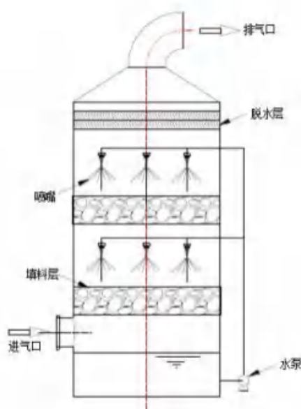
图 8.2-7 酸雾废气喷淋塔示意图
