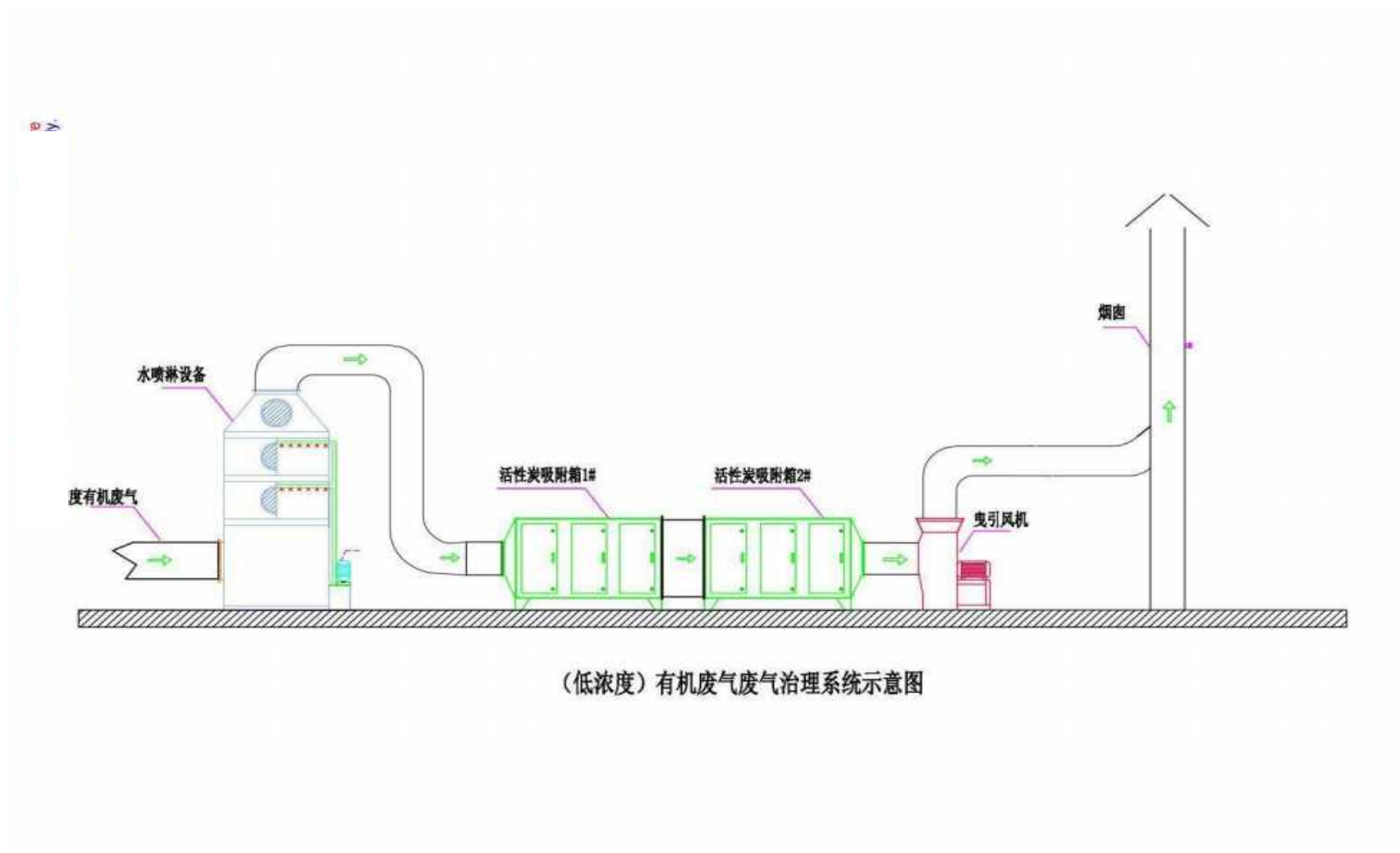
图 3.1-13 本项目低浓度有机废气治理工艺流程图
