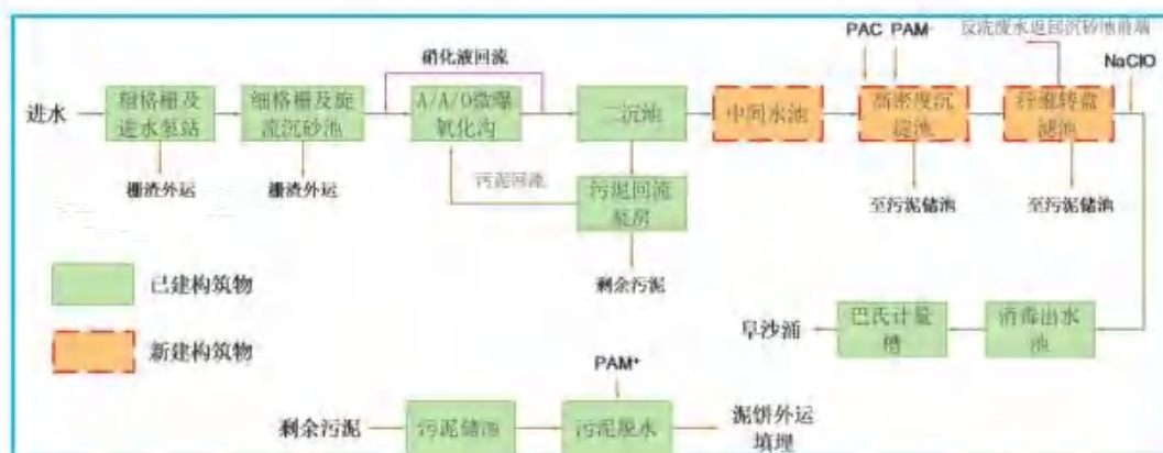
图 8.2-2 中山市阜沙镇污水处理有限公司一期、二期污水处理工艺
