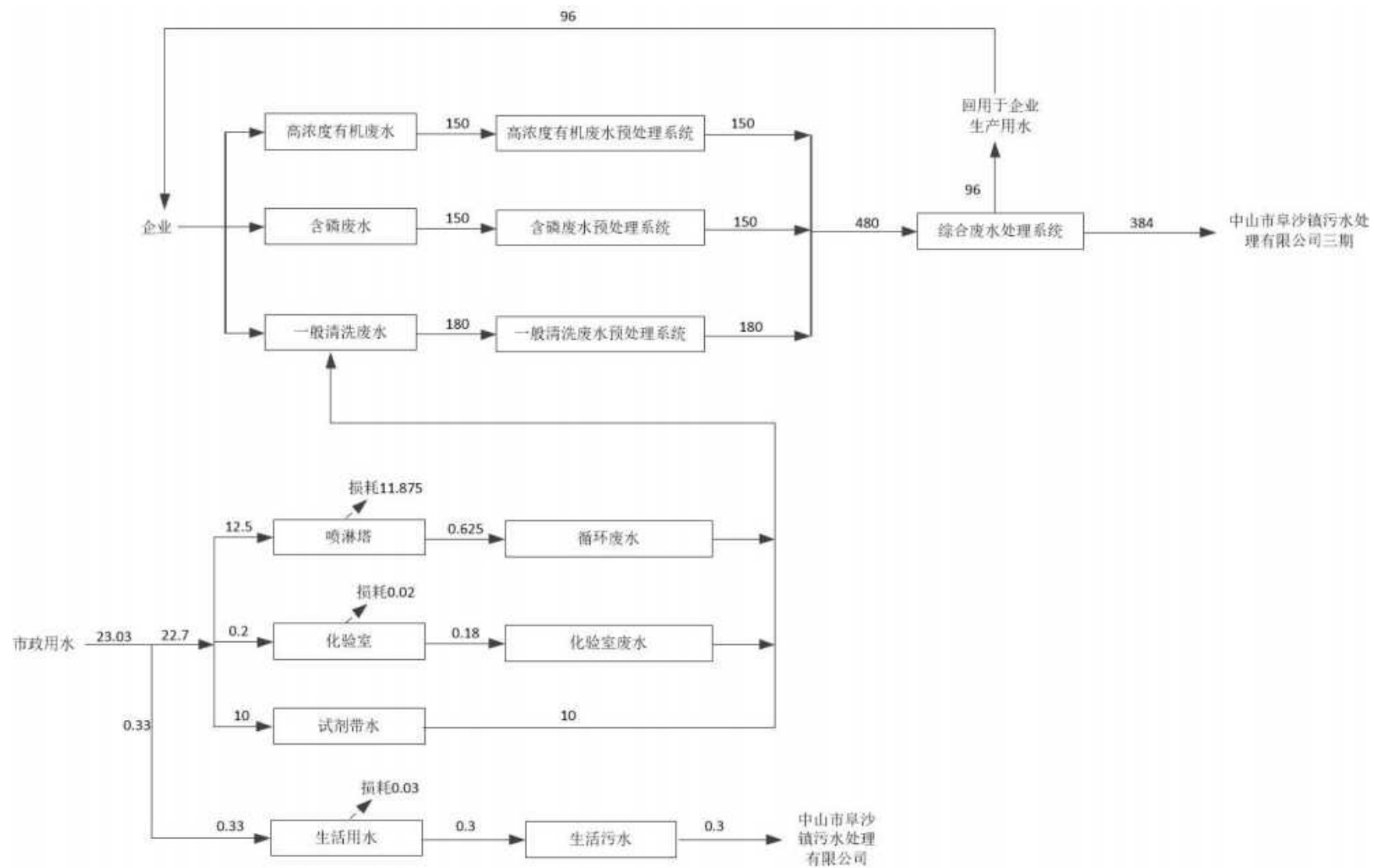
图 3.1-5 项目水平衡图 单位: \text{m}^3/\text{d}
