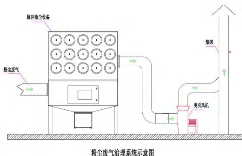
图 8.2-8 粉尘废气治理工艺流程图
