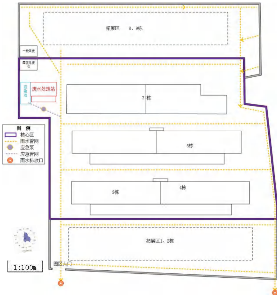
图 3.1-3 产业园雨水管网走向图
