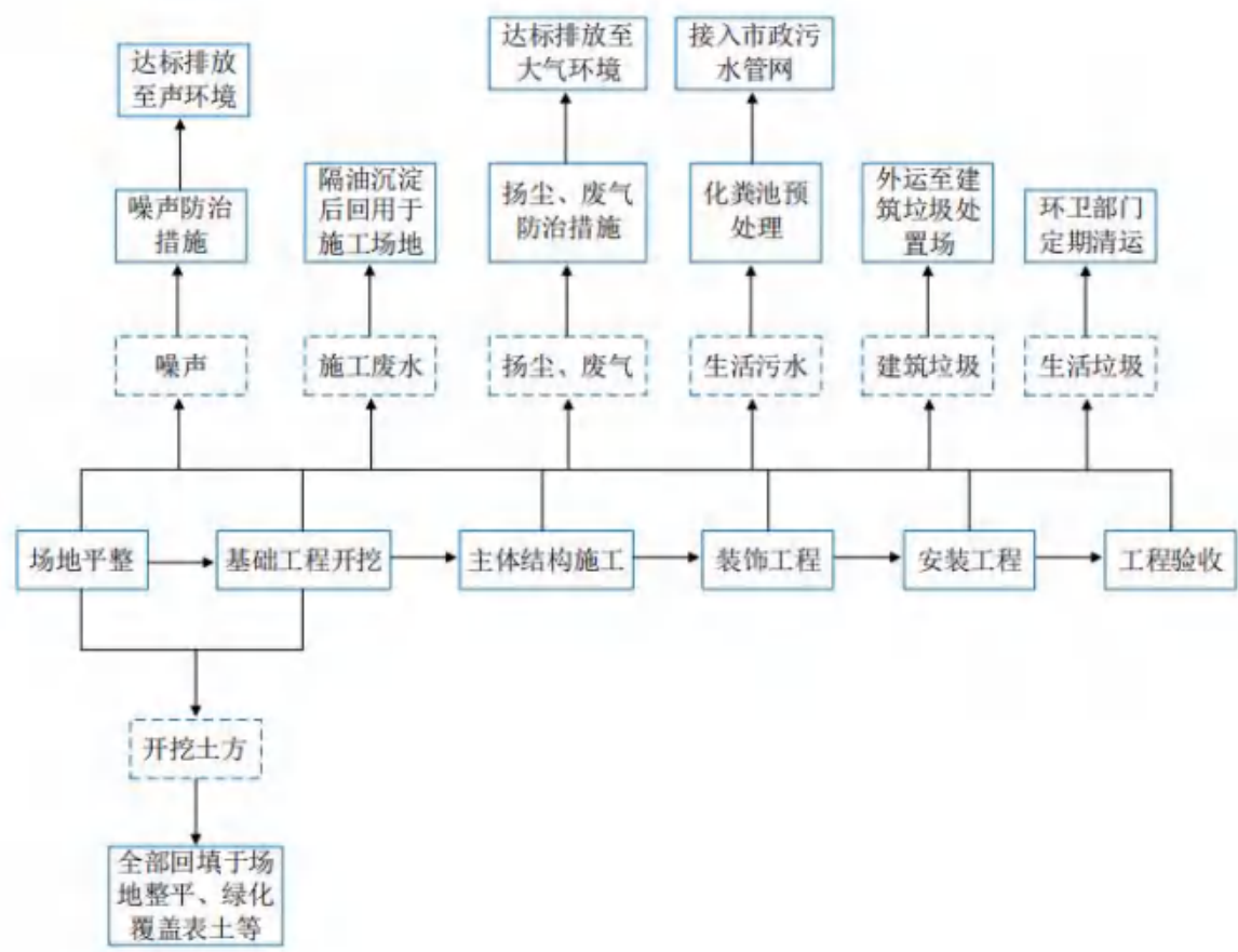
图 3.2-1 本项目施工期工艺流程及产排污环节示意图
