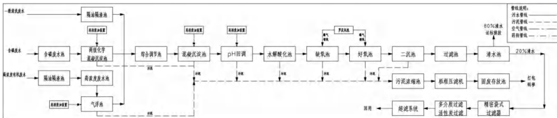
图 3.1-11 废水处理工艺流程图
