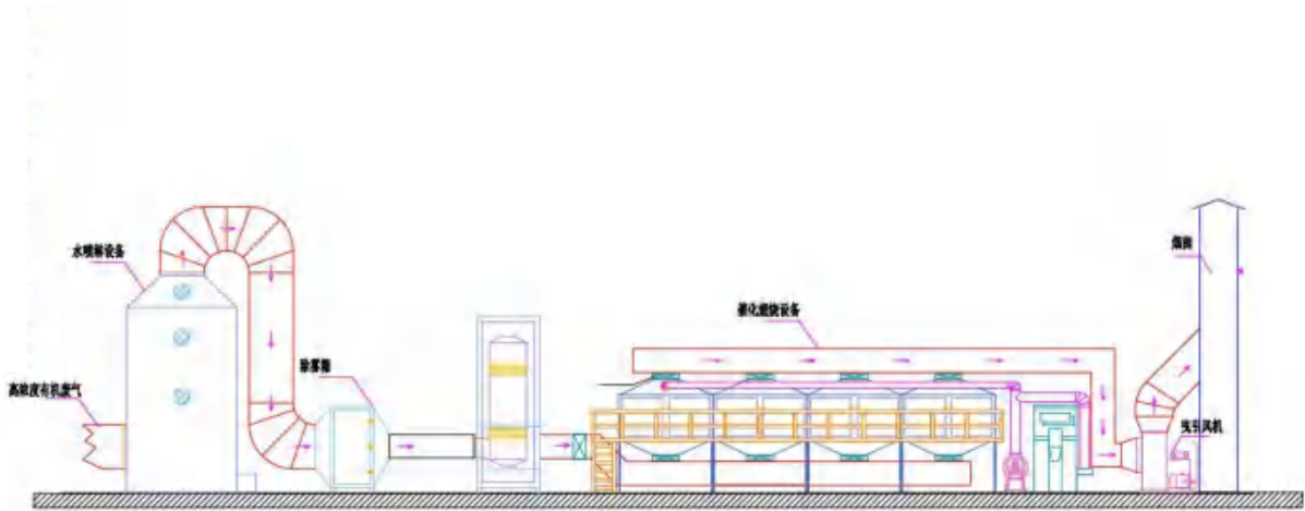
图 8.2-4 本项目高浓度有机废气治理工艺流程图
