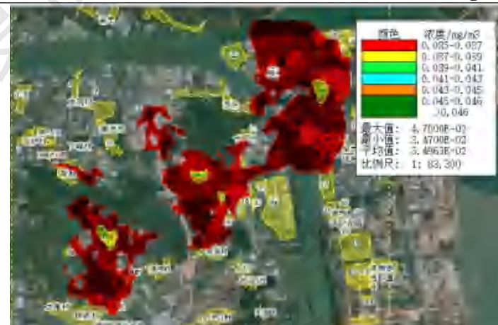
本项目 NO 2 年均浓度叠加已批在建源预测图 (单位: mg/m 3 )
