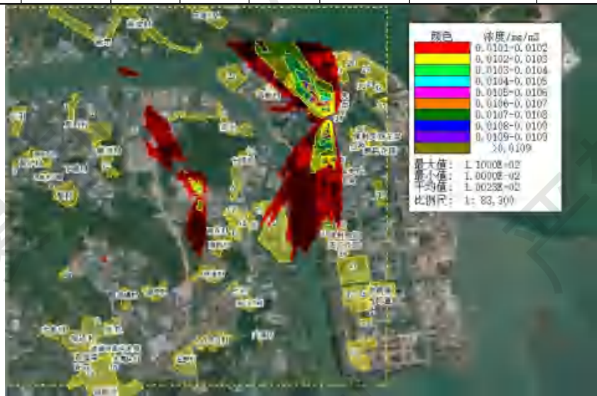
本项目 SO 2 98%保证率日均浓度叠加已批在建源预测图 (单位: mg/m 3 )
