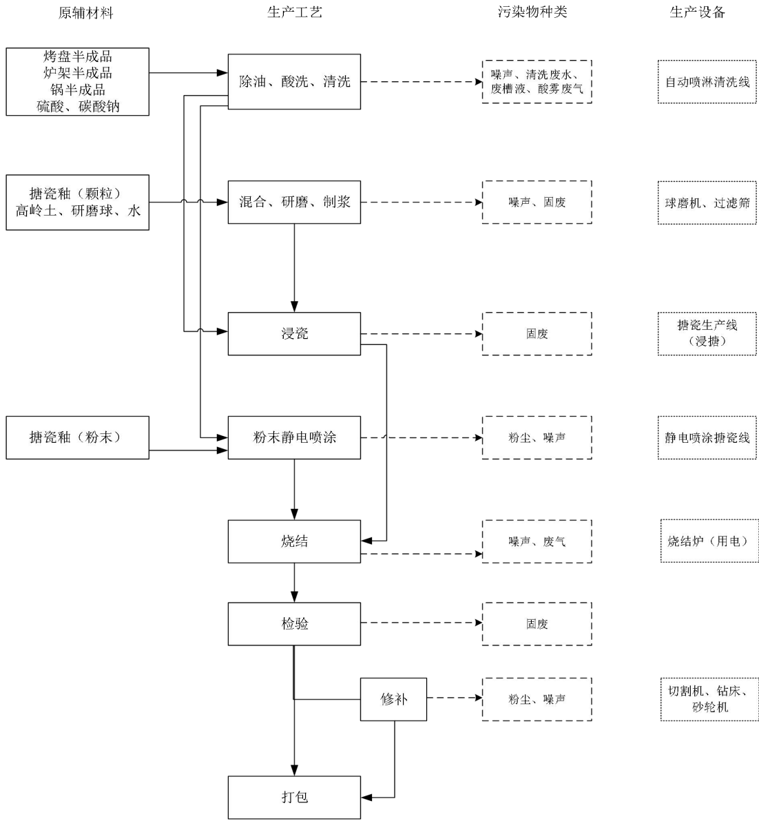
图 2 生产工艺流程图及产污环节图
