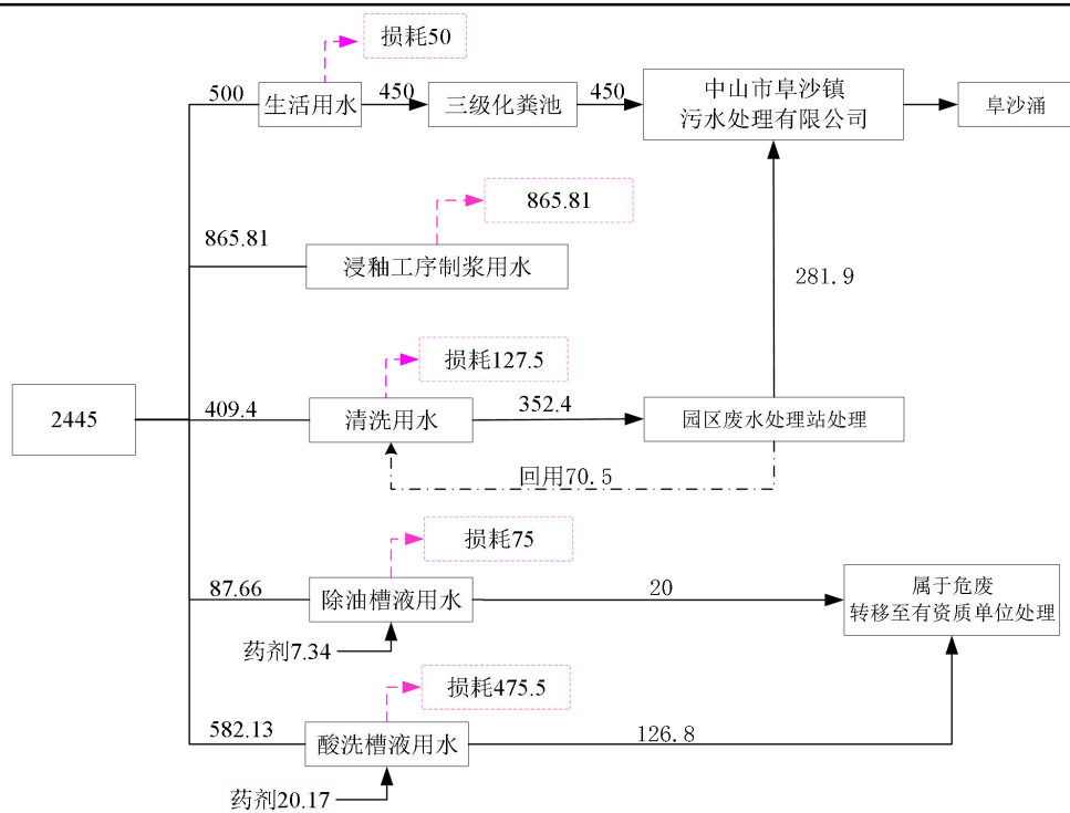
图 2-1 项目水平衡表 (m³/a)
