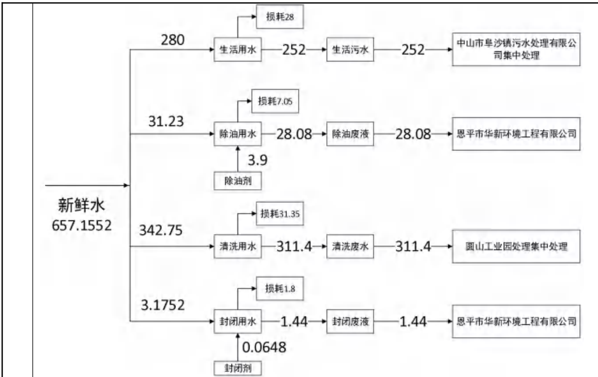
图 1 扩建前用水平衡图 (t/a)
